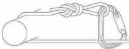
Рисунок 22. «Карабинная удавка»
